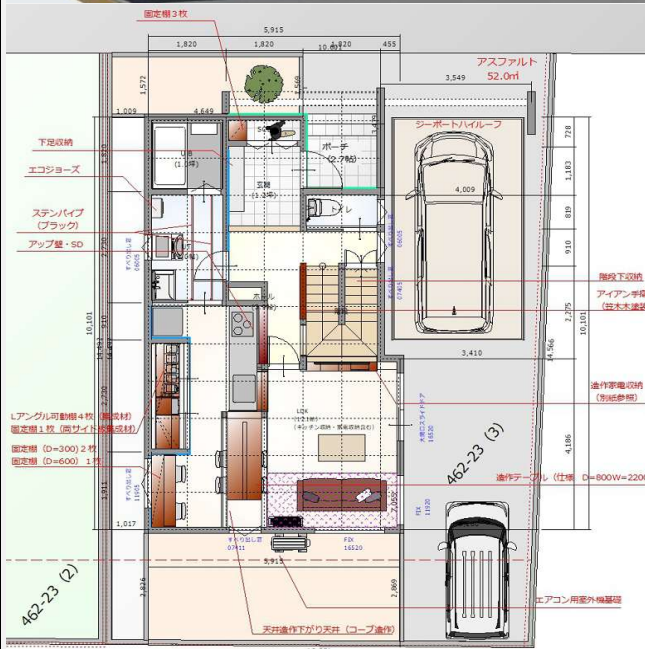
1階平面図
